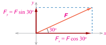
الشكل (26): المركبة الأفقية، والمركبة العمودية للمُنتَجِعِ F.
