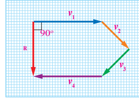
الشكل (20): محصلة السرعة.
